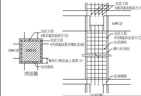
RC包覆強度補強工法
