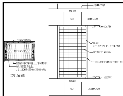
RC包覆韌性補強工法
